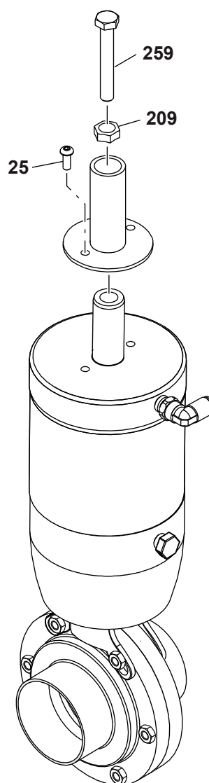
Limitador de carrera del perno en salida
