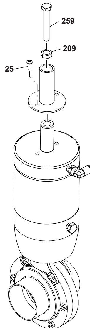
Ausgangsseitiger Hubbegrenzer
