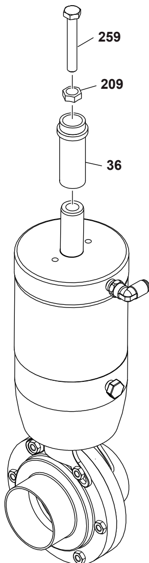
Eingangsseitiger Hubbegrenzer
