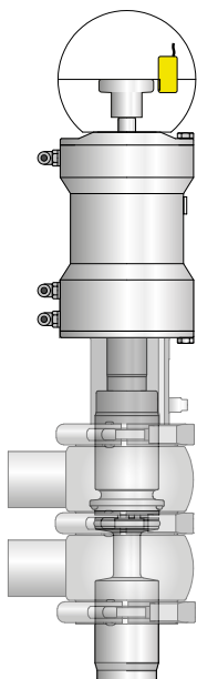
Vanne fermée
