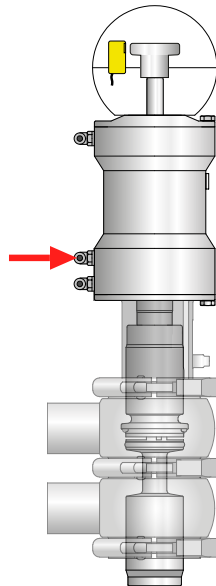
Åben ventil
