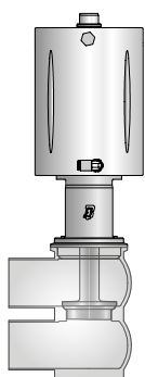
Normalement fermée
